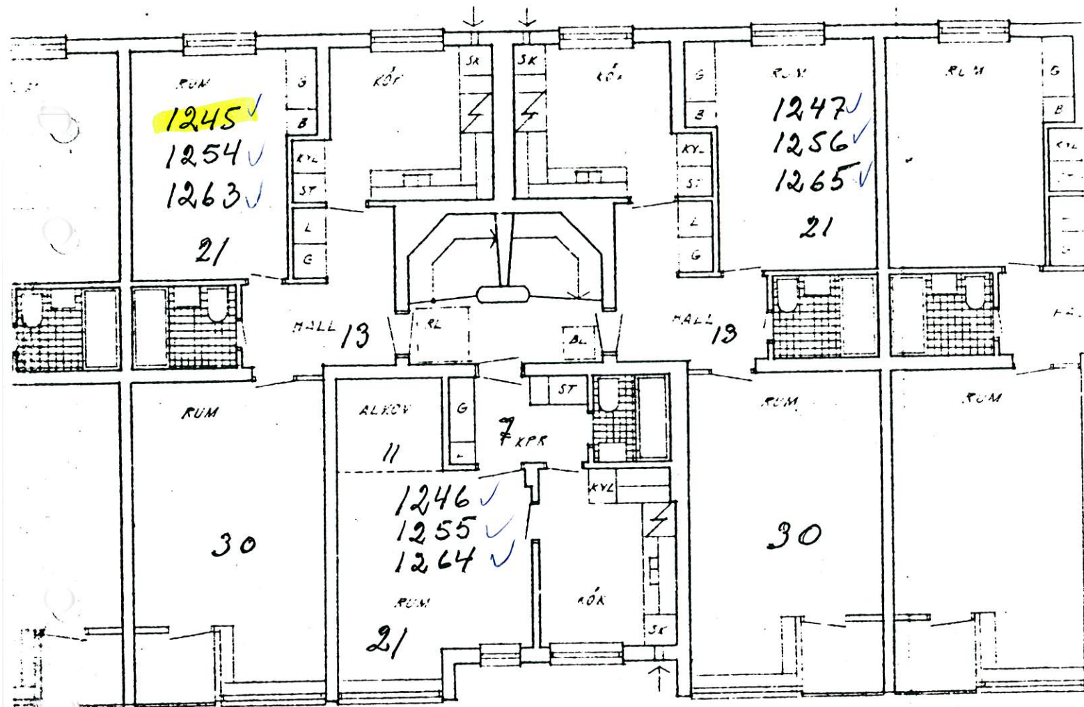
VÅNINGSPLAN
