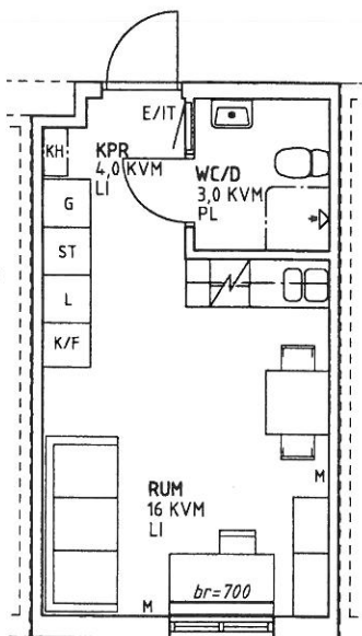
LÄGENHETSPLAN
