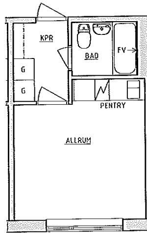
1ROK LÄGENHET TYP1-A
