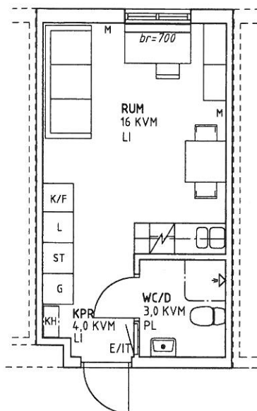
LÄGENHETSPLAN
