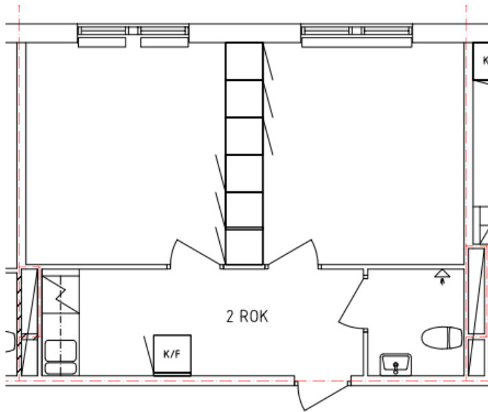
Ritning 2 rum och kokvrå, 38 kvm, Röntgenvägen 5
