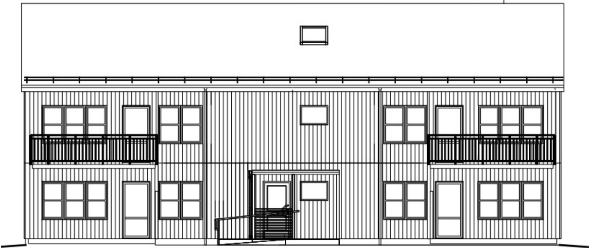
FASAD 1
