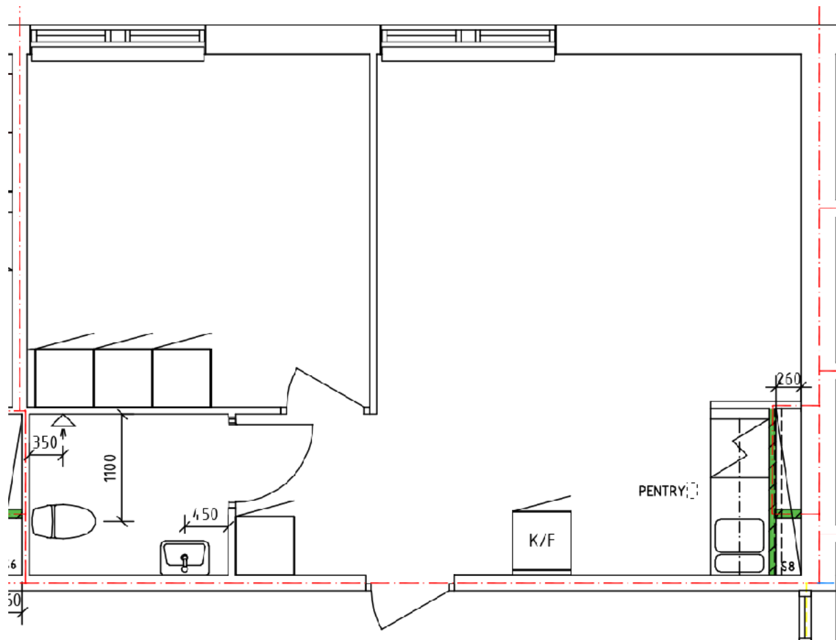
Ritning 2 rum och kokvrå, 42 kvm, öppen planlösning, Röntgenvägen 5
